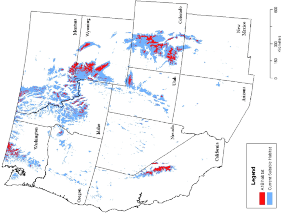
A1B Scenario
