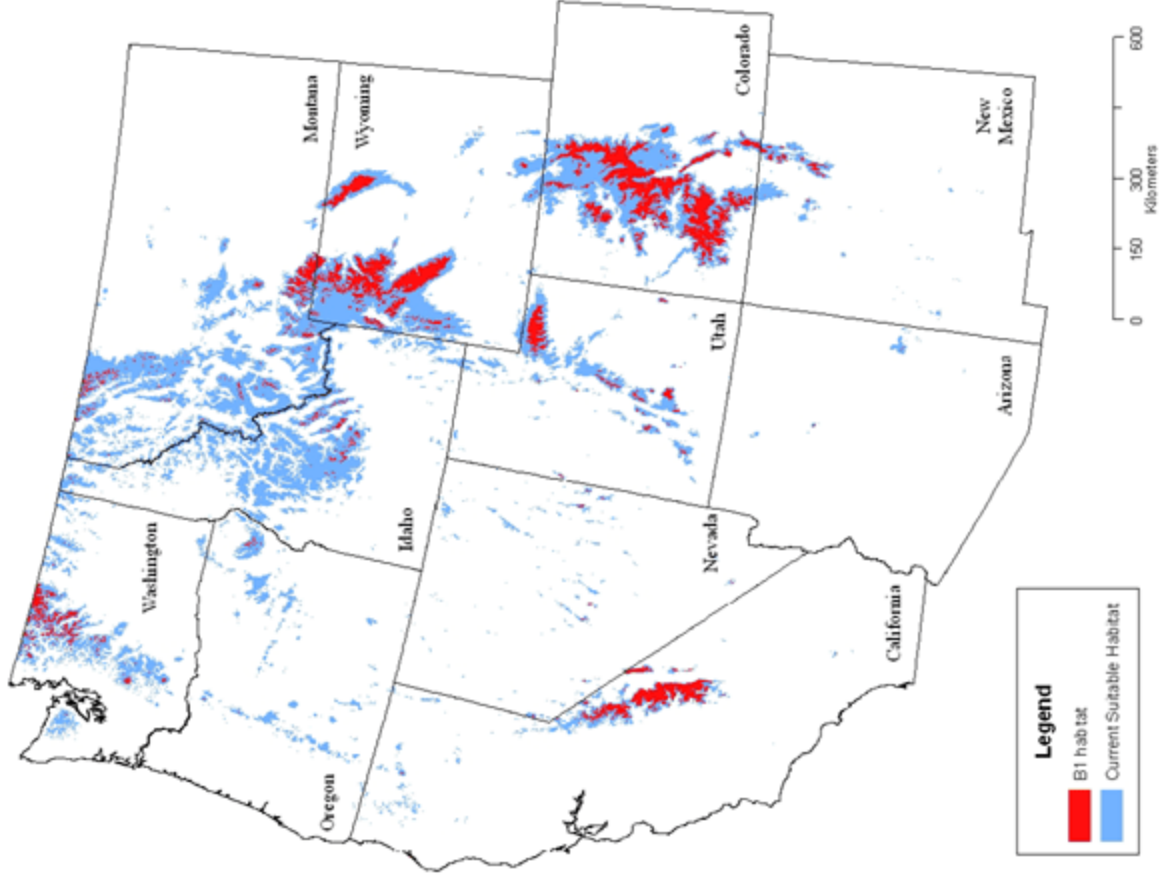
B1 Scenario
