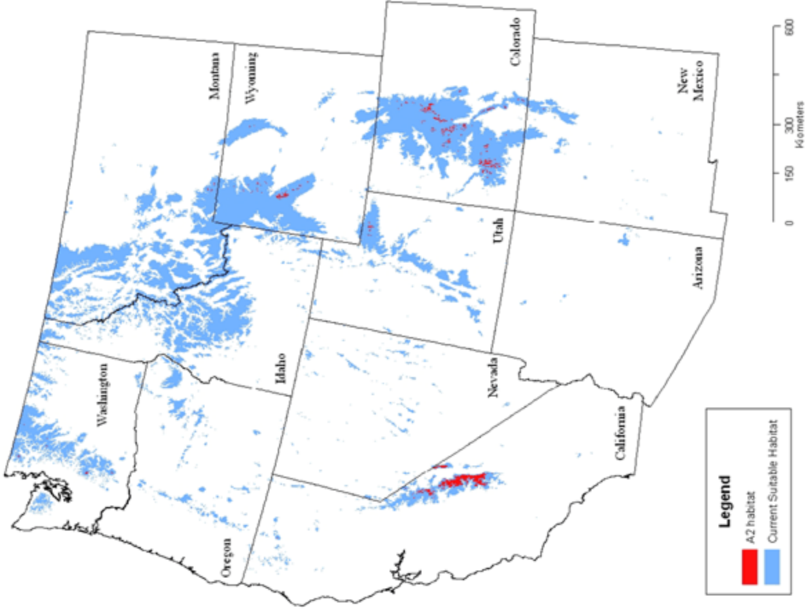
A2 Scenario
